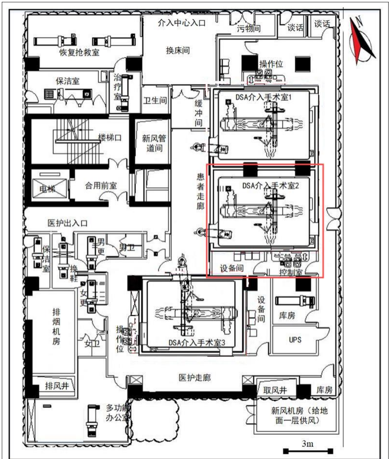
图 2-3 介入手术室平面布置图
