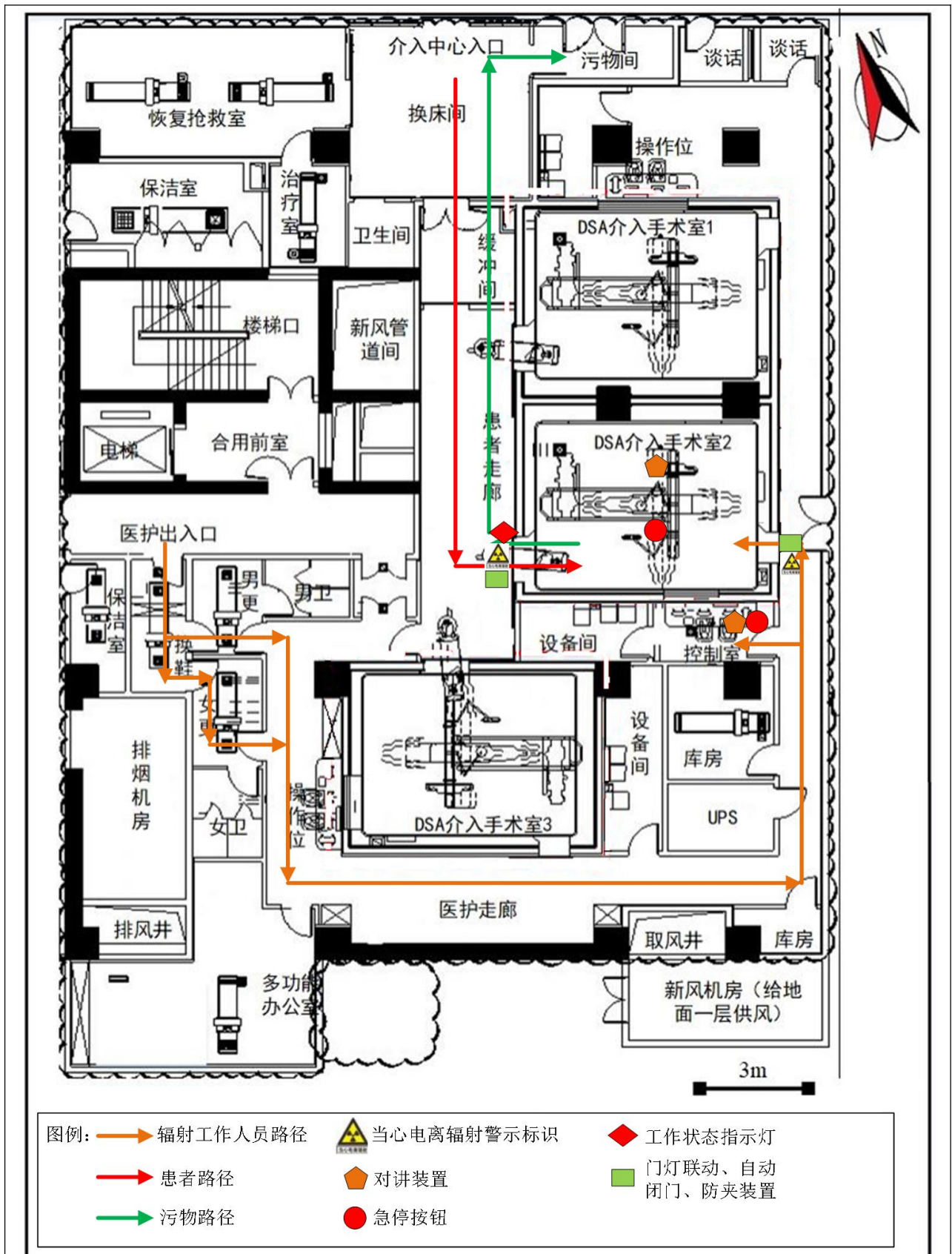
图 3-2 辐射工作人员、患者、污物流动路线图和辐射安全设施安装位置示意图
