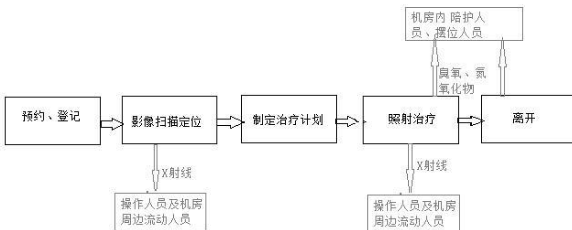
图2-5 射波刀污染物及污染途径示意图
