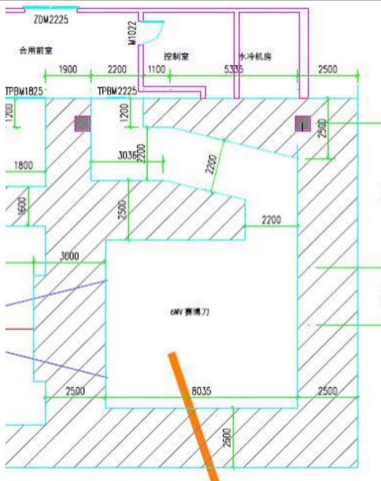
图2-3 射波刀治疗室机房设计布局图
